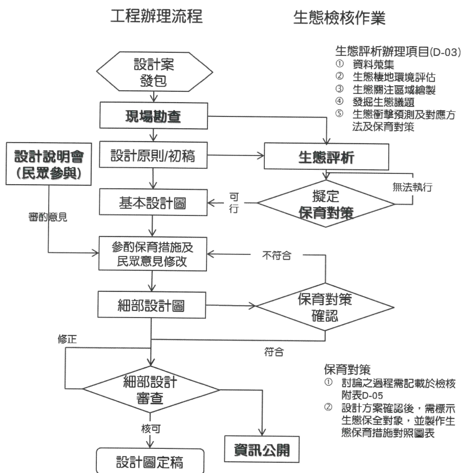
圖 2-1 規劃設計階段生態檢核作業流程圖
