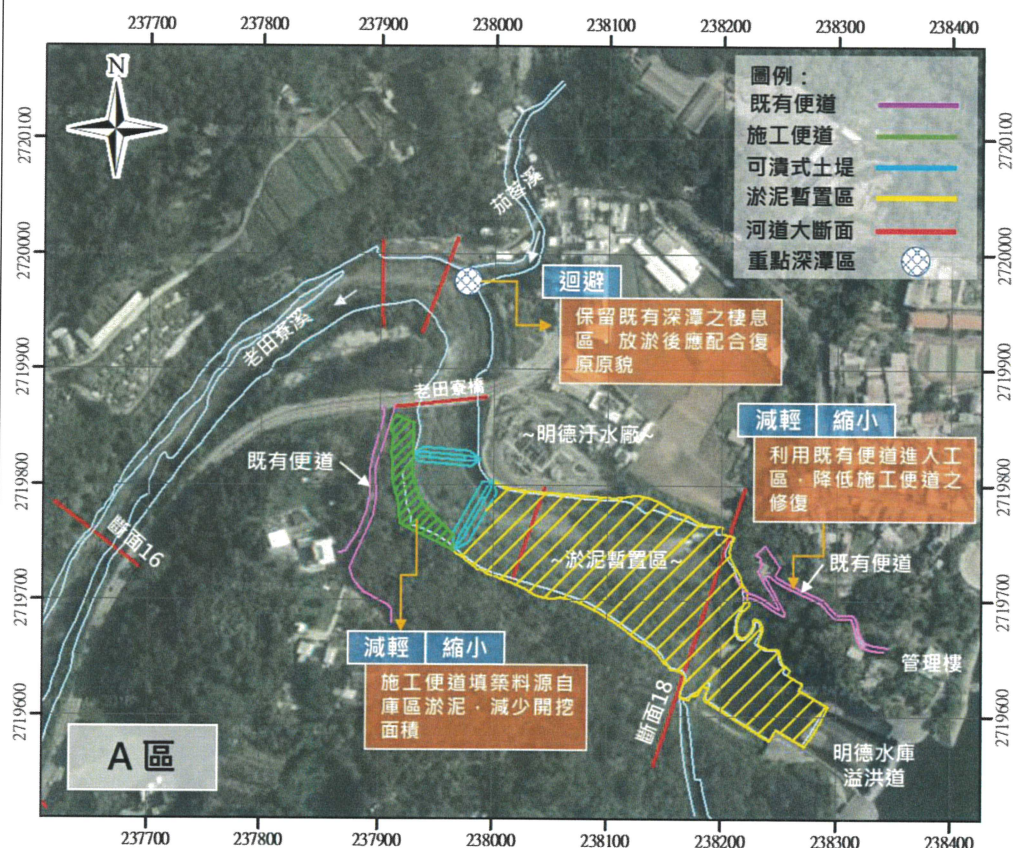
生態保育措施平面圖：
