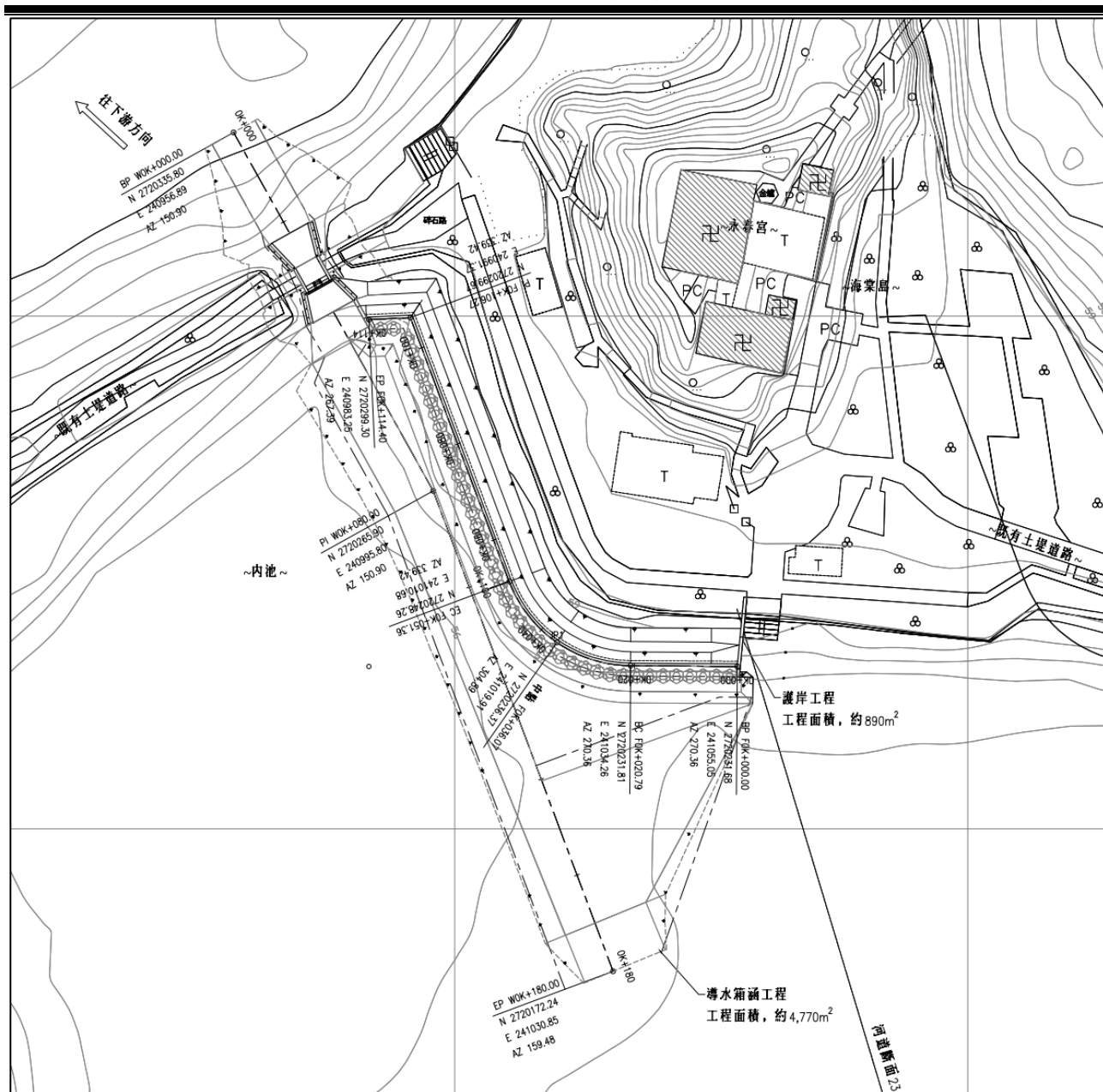
圖 1-1 明德水庫海棠島內池清淤工程(陸挖)及護岸改善工程平面配置圖
